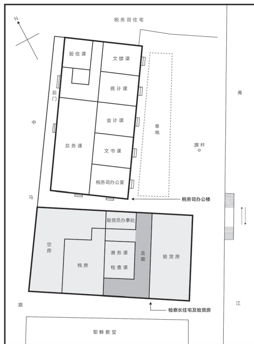
图9 检察长住宅及验货房首层平面简图(北侧为税务司办公楼) (作者重绘,底图来自任与孝.宁波海关志[M].杭州:浙江科学技术出版社,2000.)
