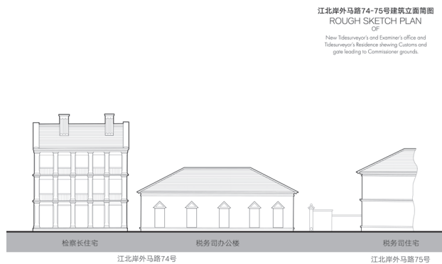
图6 江北岸74~75地块建筑立面简图(从左至右依次为: 检察长住宅、税务司办公楼、税务司住宅) (作者重绘, 底图由浙海关旧址博物馆提供)
